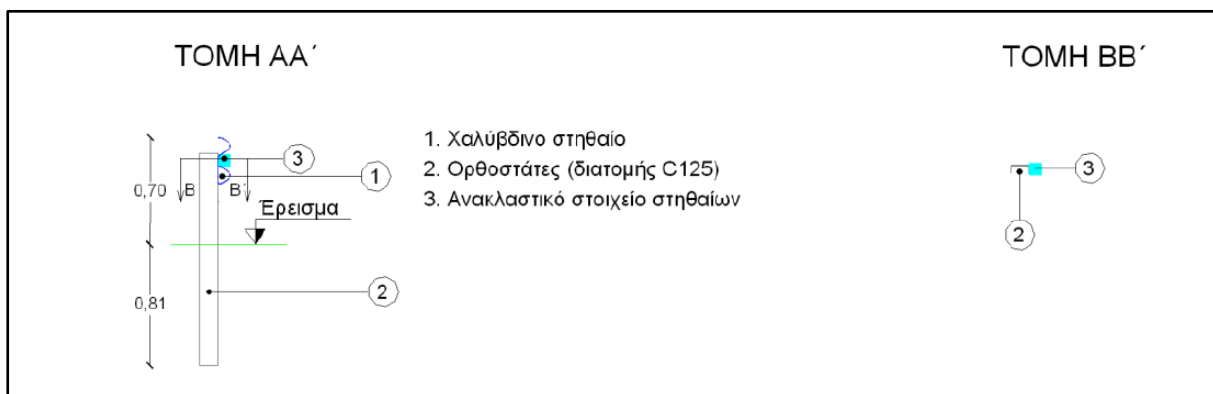
Σχ. 3: Μονόπλευρο χαλύβδινο στηθαίο ασφαλείας (το σχήμα είναι άνευ κλίμακας).
